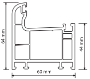
W 6310 Kasa Profili Frame Profile Ağırlık / Weight : 0.870 kg / mt
