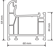
W 6410 Kasa Profili / Frame Profile Ağırlık / Weight : 0.955 kg/mt
