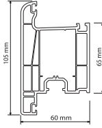
W 6450 Dışa Açılan Kapı Kanat Profili Reverse Door Sash Profile Ağırlık / Weight : 1.400 kg / mt
