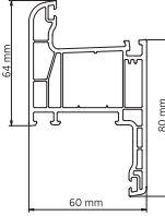
W 6410 P Pervazlı Kasa Profili Border Frame Profile Ağırlık / Weight : 1.260 kg / mt
