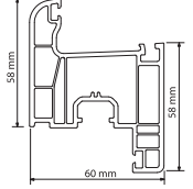
W 6420 Kanat Profili / Sash Profile Ağırlık / Weight : 1.080 kg/mt
