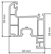
W 6320 Kanat Profili Sash Profile Ağırlık / Weight : 1.010 kg / mt
