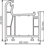
W 6410 S Süper Kasa Profili Super Frame Profile Ağırlık / Weight : 1.100 kg / mt
