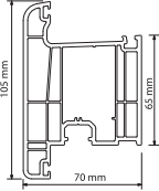
W 7050 Dışa Açılan Kapı Kanat Profili Reverse Door Sash Ağırlık / Weight : 1.550 kg/mt
