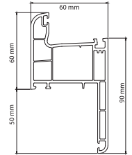
W 6310P Pervazlı Kasa Profili Border Frame Profile Ağırlık / Weight : 1.140 kg/mt
