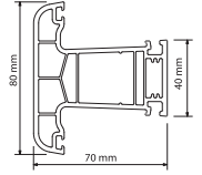
W 7030 Orta Kayıt Profili Mullion Profile Ağırlık / Weight : 1.170 kg/mt
