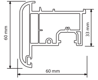
W 6460 Hareketli Orta Kayıt Profili Moveable Mullion Profile Ağırlık / Weight : 0.872 kg / mt
