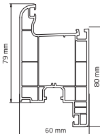
V 6440 Kapı Kanat Profili Door Sash Profile Ağırlık / Weight : 1.213 kg / mt
