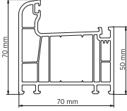
W 7010 S Süper Kasa Profili Super Frame Profile Ağırlık / Weight : 1.180 kg/mt
