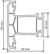
W 6430 Orta Kayıt Profili Mullion Profile Ağırlık / Weight : 1.010 kg / mt
