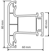
W 6330 Orta Kayıt Profili Sash Profile Ağırlık / Weight : 0.930 kg / mt
