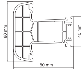
W 8030 Orta Kayıt Profili / Mullion Profile Ağırlık / Weight: 1.420 kg / mt
