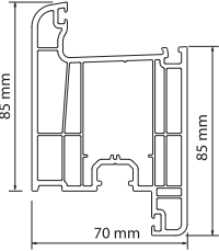
W 7040 Kapı Kanat Profili Door Sash Profile Ağırlık / Weight: 1.700 kg / mt
