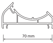
W 7120 70 mm Köşe Dönüş Adaptörü 70 mm Corner Turning Adapter Ağırlık / Weight : 0.605 kg / mt
