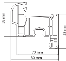
W 8020 Damlalıklı Kanat Profili Self Drainage Sash Profile Ağırlık / Weight: 1.400 kg / mt
