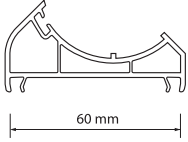
W 6520 60 mm Köşe Dönüş Adaptörü 60 mm Corner Turning Adapter Ağırlık / Weight : 0.520 kg / mt
