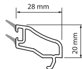
W 7080 Çift Cam Çıtası (20 mm) Double Glass Bead (20 mm) Ağırlık / Weight: 0.240 kg / mt
