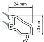
W 7070 Çift Cam Çıtası (24 mm) Double Glass Bead (24 mm) Ağırlık / Weight: 0.225 kg / mt
