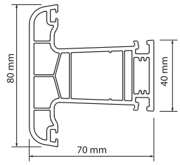
W 7030 Orta Kayıt Profili Mullion Profile Ağırlık / Weight: 1.250 kg / mt
