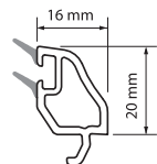
W 6470 Üç Cam Çıtası (32 mm) Three Glass Bead (32 mm) Ağırlık / Weight: 0.180 kg / mt
