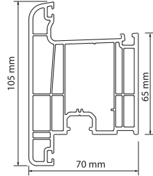
W 7050 Dışa Açılan Kapı Kanat Profili Reverse Door Sash Ağırlık / Weight: 1.700 kg / mt
