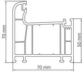
W 7010 S Süper Kasa Profili Super Frame Profile Ağırlık / Weight: 1.230 kg / mt
