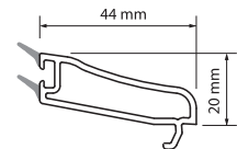
W 7090 Tek Cam Çıtası (4 mm) Single Glass Bead (4 mm) Ağırlık / Weight: 0.310 kg / mt
