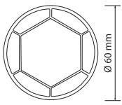
W 7110 Köşe Dönüş Borusu Corner Turning Pipe Ağırlık / Weight : 0.745 kg / mt
