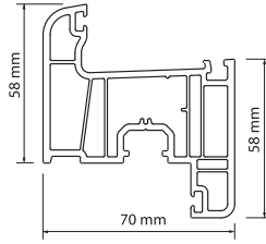
W 7020 Kanat Profili / Sash Profile Ağırlık / Weight: 1.300 kg / mt
