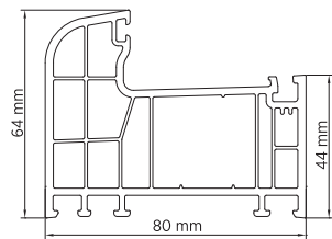
W 8010 Kasa Profili / Frame Profile Ağırlık / Weight: 1.310 kg / mt
