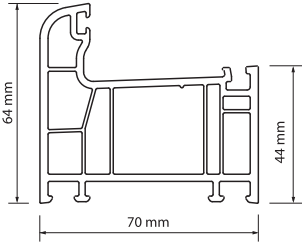
W 7010 Kasa Profili / Frame Profile Ağırlık / Weight: 1.160 kg / mt
