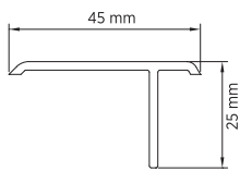
W 9040 T Kapama Asymmetrical T Ağırlık / Weight : 0.200 kg / mt
