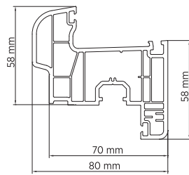
W 8020 Damlalıklı Kanat Profili Self Drainage Sash Profile Ağırlık / Weight: 1.400 kg / mt
