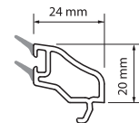
W 7070 Çift Cam Çıtası (24 mm) Double Glass Bead (24 mm) Ağırlık / Weight: 0.225 kg / mt
