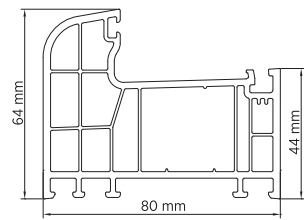
W 8010 Kasa Profili / Frame Profile Ağırlık / Weight: 1.310 kg / mt
